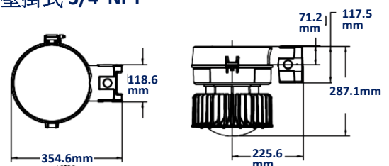
壁掛式 3/4"NPT
