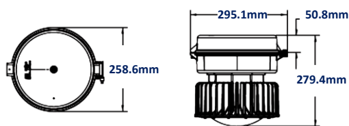
吊管式 3/4"NPT
