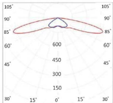
對稱長方形燈光分佈
