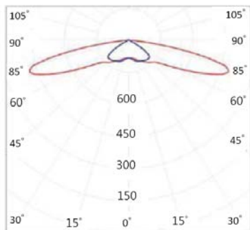
對稱長方形燈光分佈
