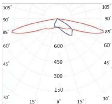
不對稱長方形燈光分佈
